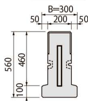
正面図
