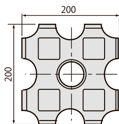
ブロックの寸法
