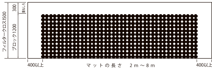
マットの寸法
