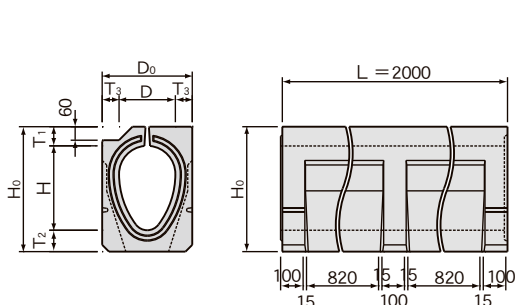
側溝製品図
