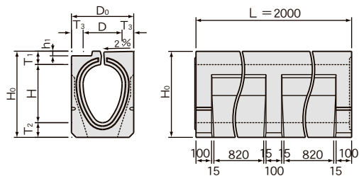
側溝製品図
