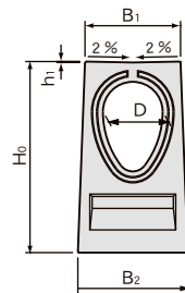
柵製品図
