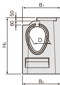
柵製品図
