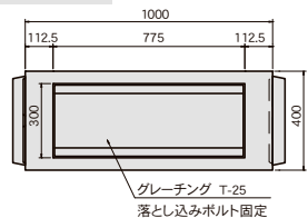
平面図
