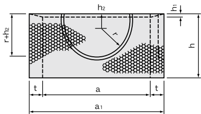
側面図 中・下
