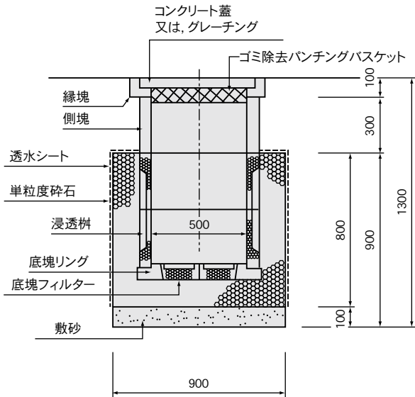
断面例 (EMBX-500)
