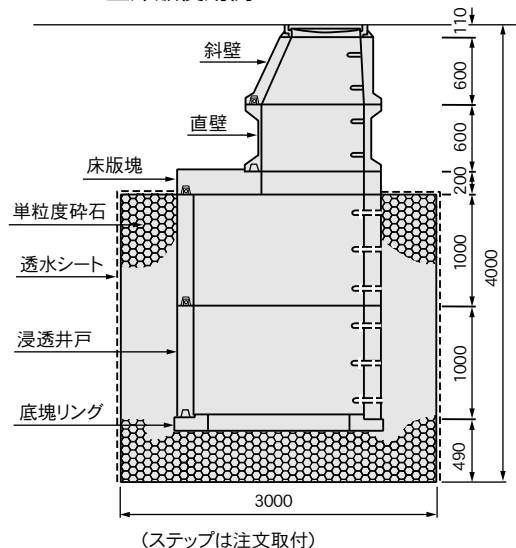
EW-1500型床版使用例
