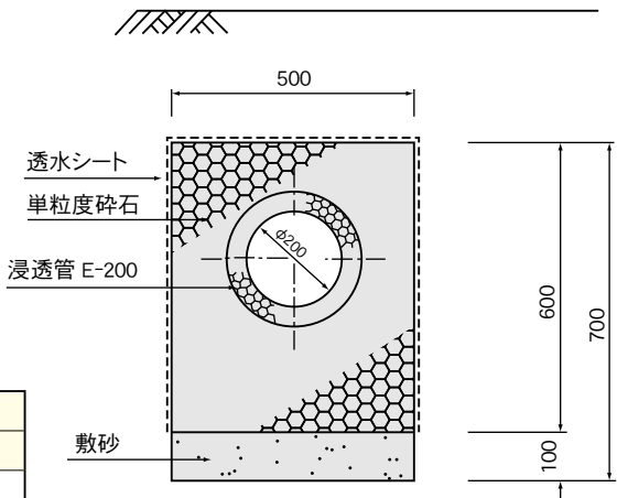
断面例 (E-200)
