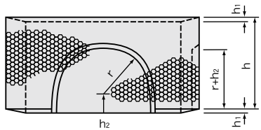
側面図 上
